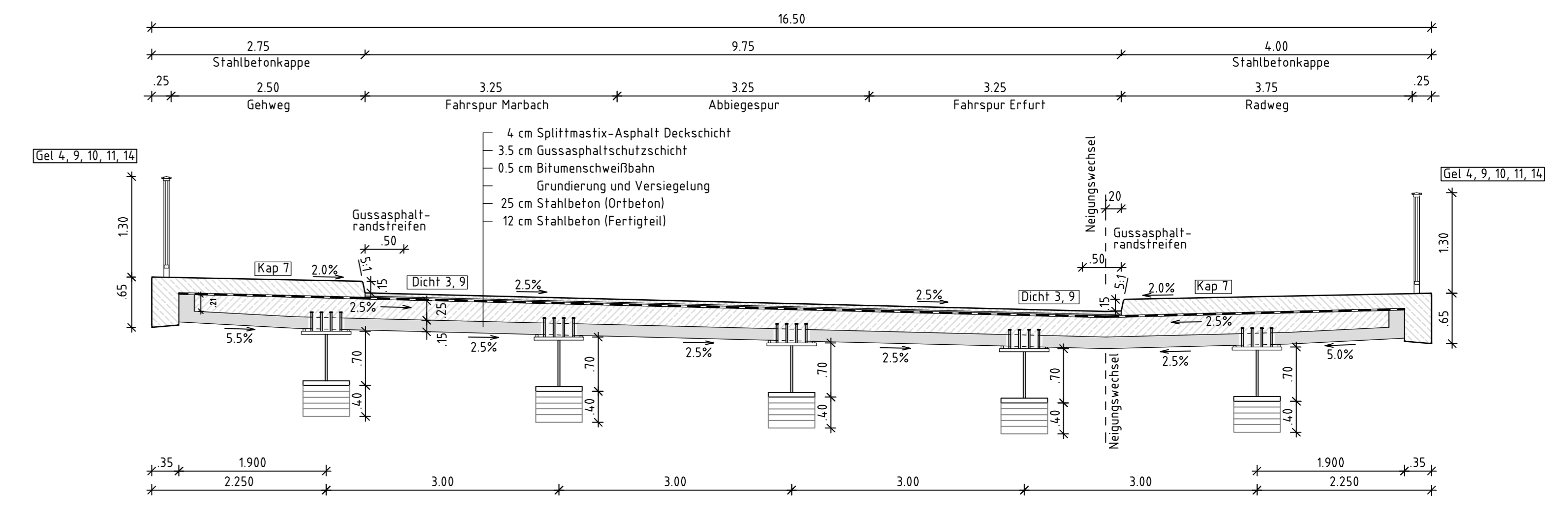
Regelquerschnitt Variante 2 - 2 Fahrspuren + Abbiegespur M 1:50
