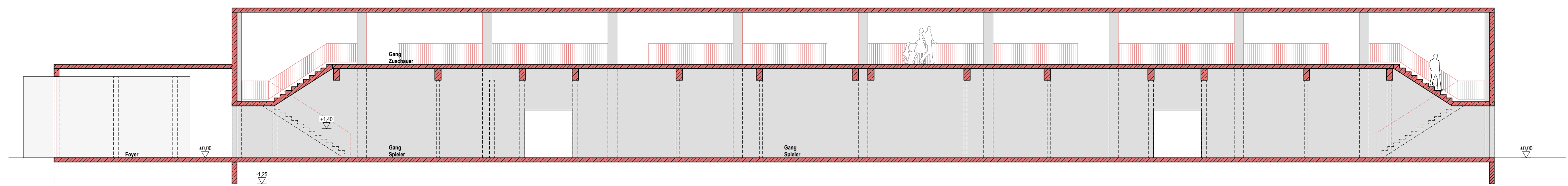
LÄNGSSCHNITT
