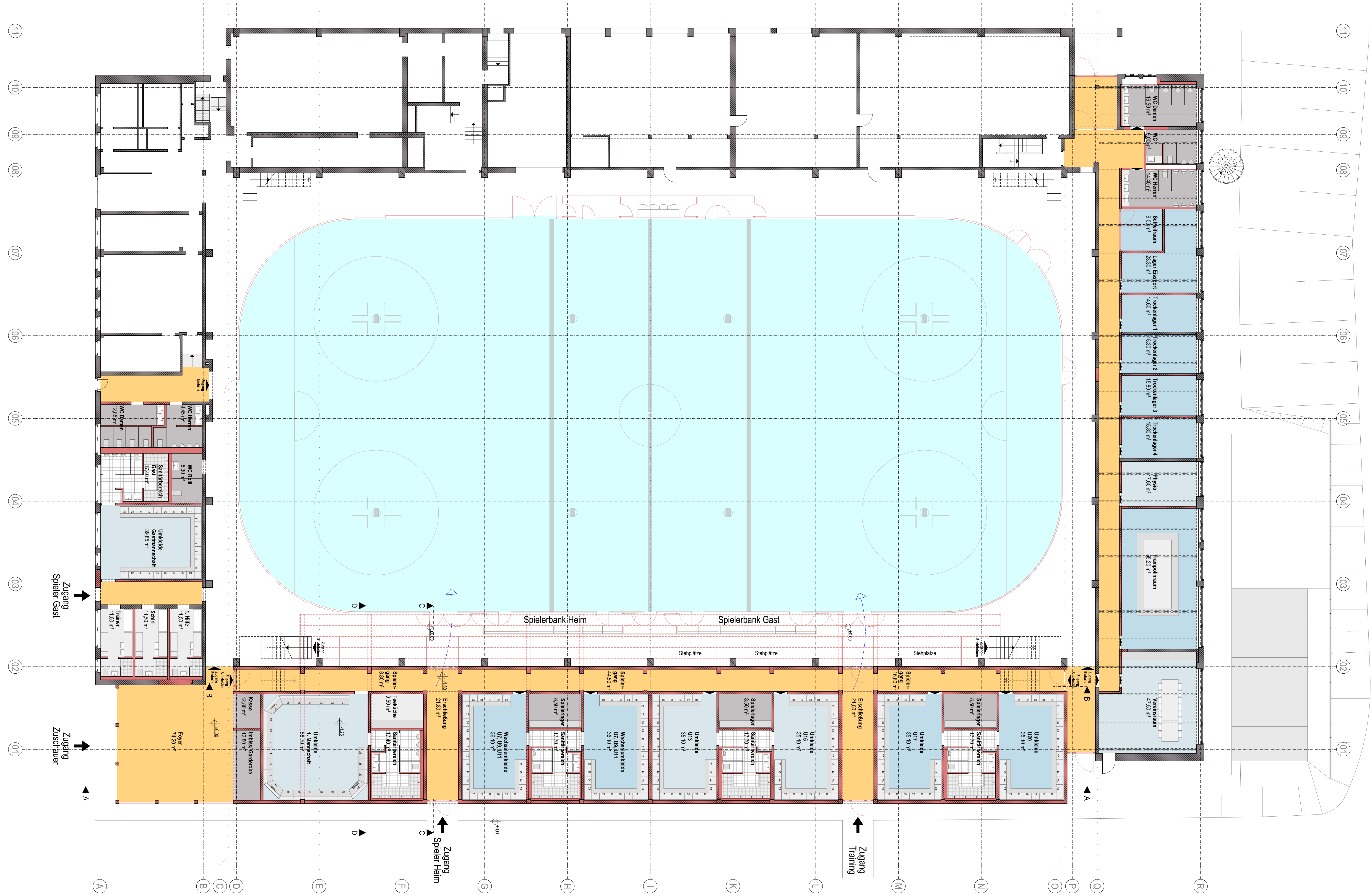
GRUNDRISS EBENE EISFLÄCHE
