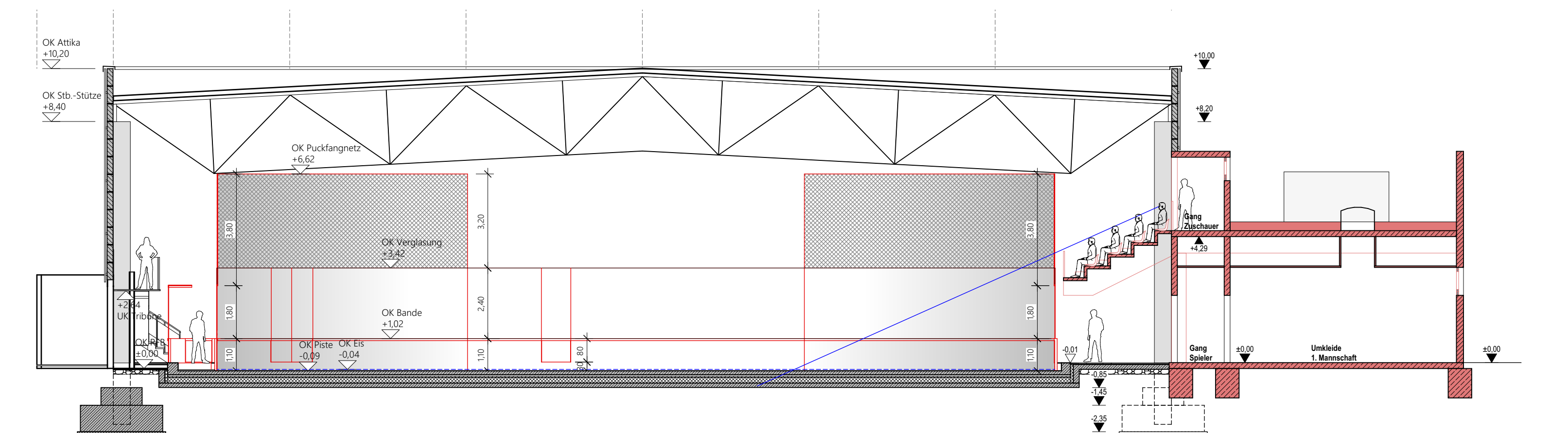
QUERSCHNITT
