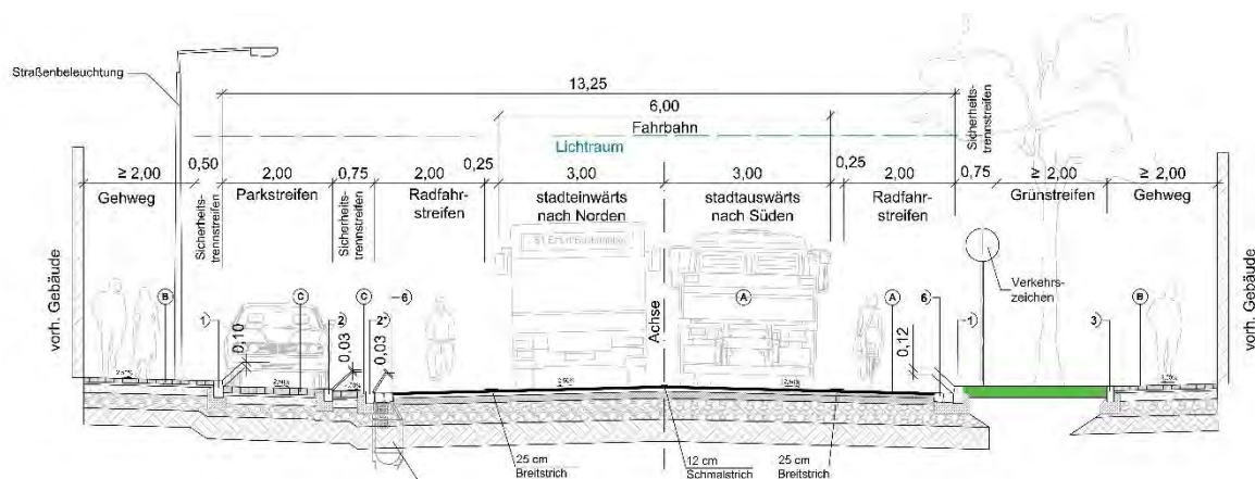
Bild 6, Regelquerschnitt
