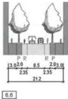
Bild 2: Auszug RASSt 06, Querschnitt 6.6
