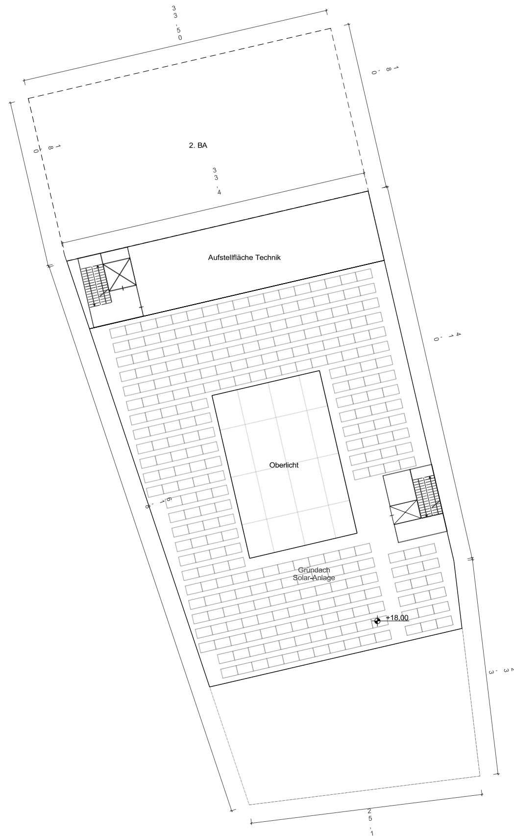
Dachgeschoss
