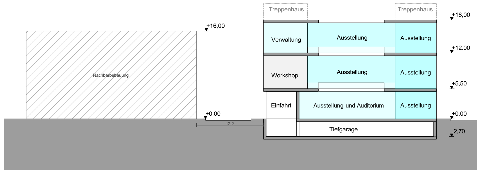
Schnitt BB
