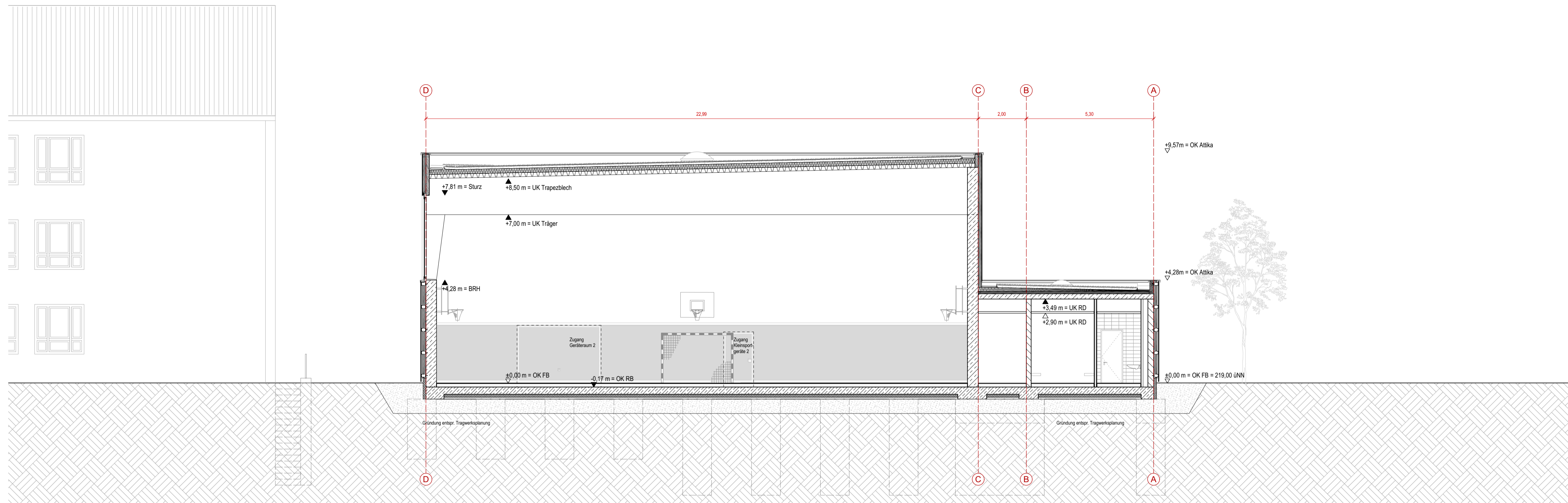
Schnitt AA
