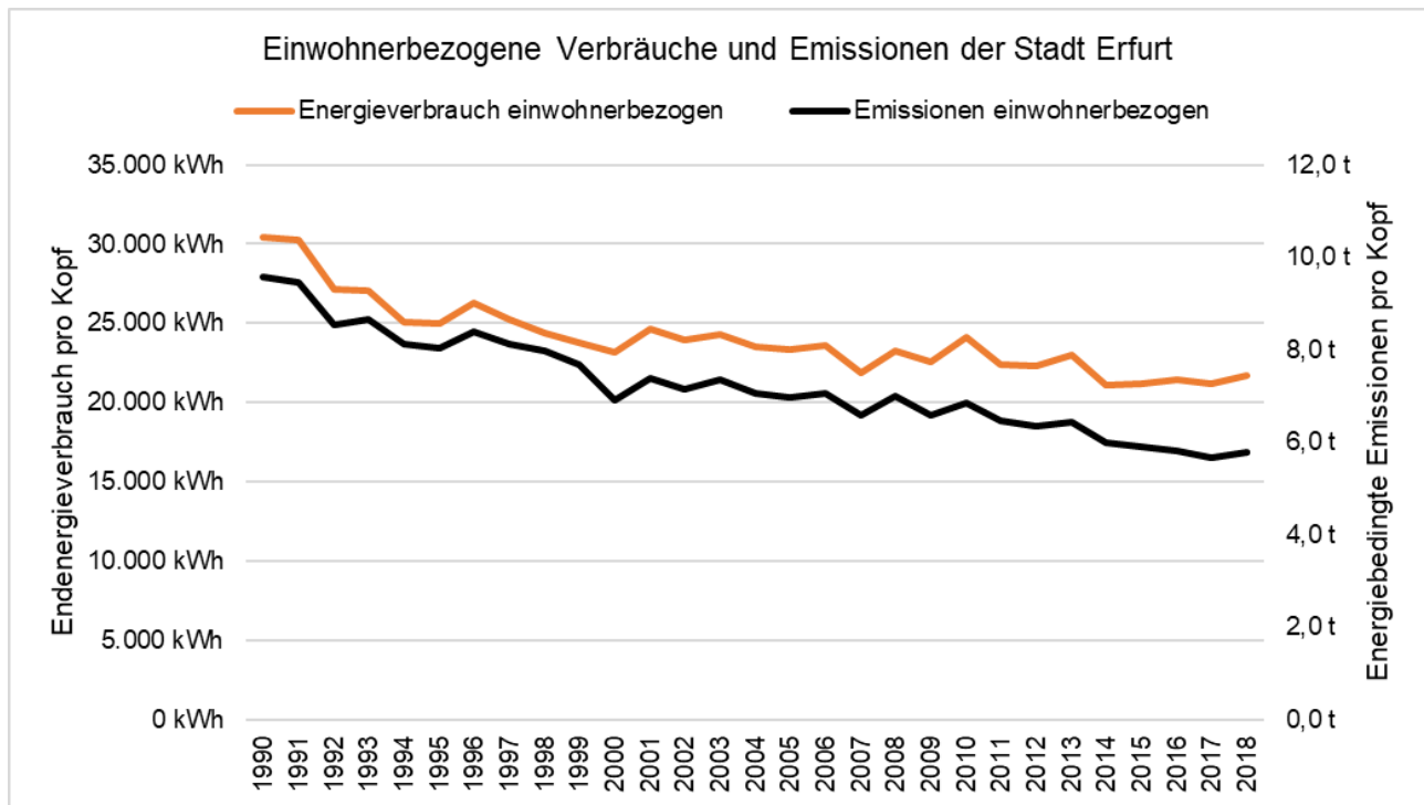
Abbildung 21: Einwohnerbezogene Verbräuche und Emissionen der Stadt Erfurt 1990 - 2018
