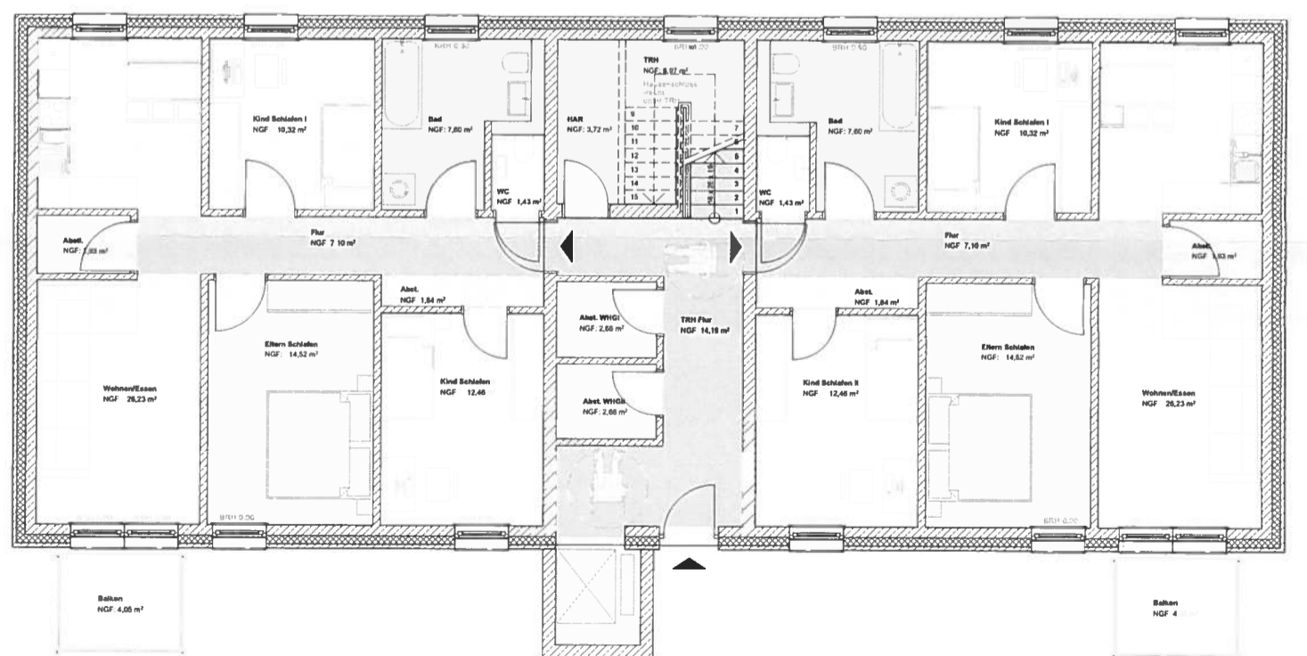
Grundriss Erdgeschoss 2 x 4-Raum Wohnung
