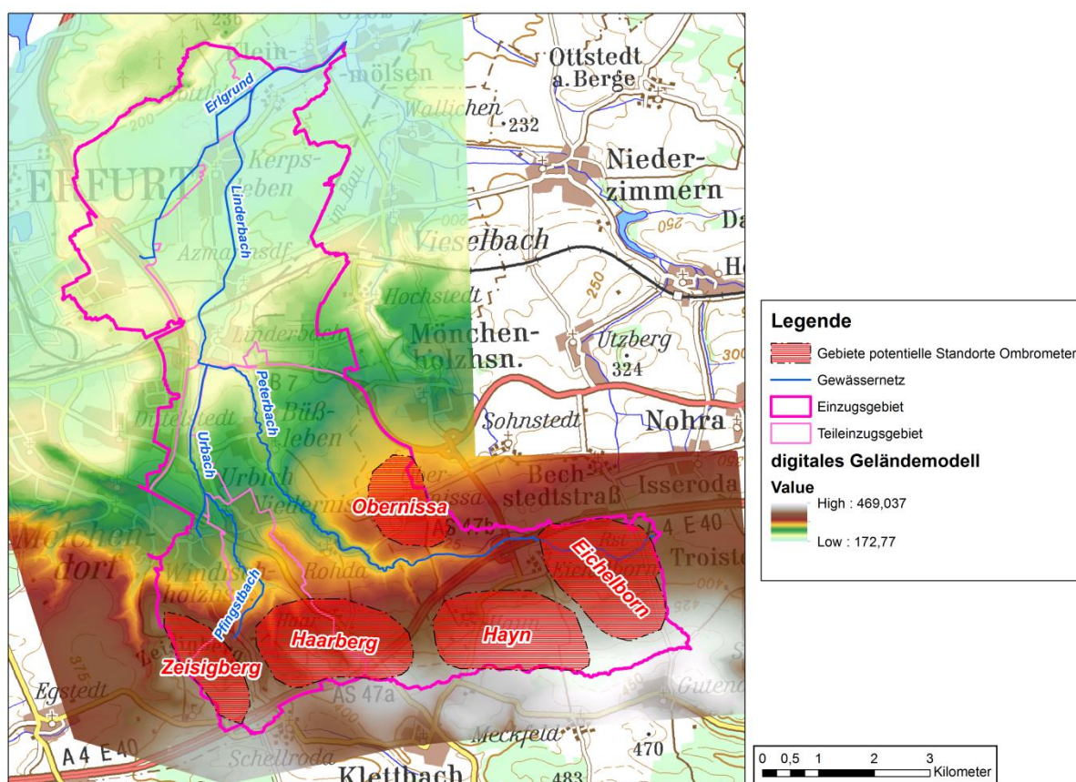
Abbildung 9-2 Identifizierte Bereiche für Ombrometerstationen zur Frühwarnung
