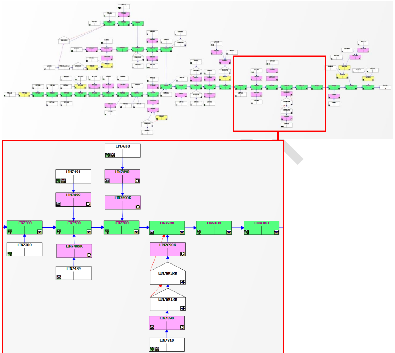
Abbildung 6-4 NASIM-Systemplan Linderbach
