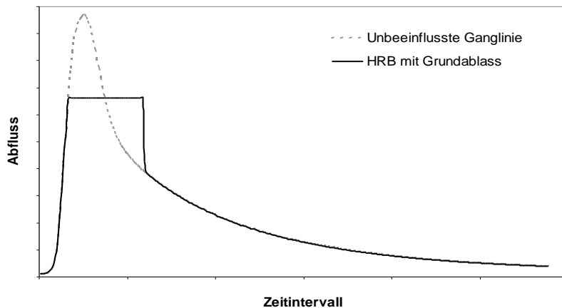
Abbildung 8-9 Wirkung eines HRB mit konstanter Abgabe über Grundablass (vereinfachte Darstellung)
