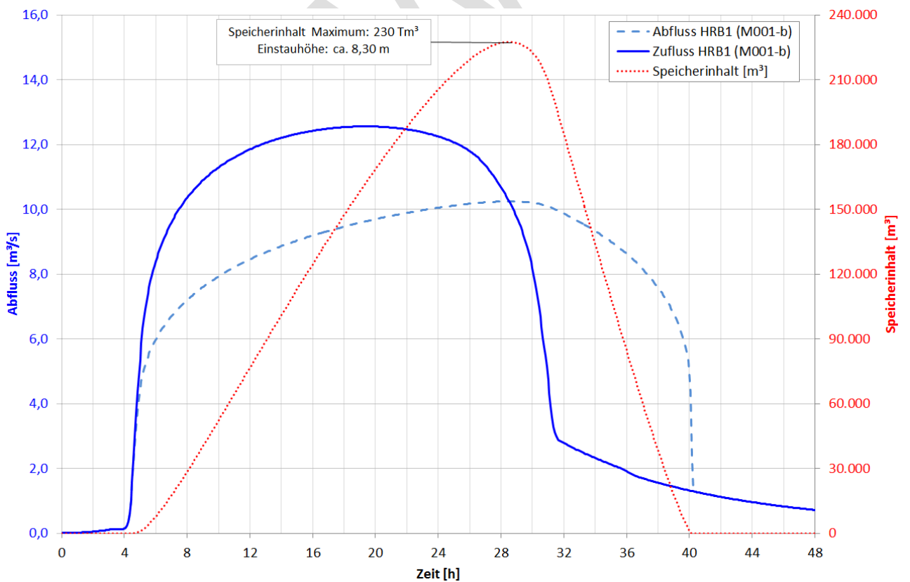
Abbildung 8-14 Variante 2: Ganglinien der Speichersimulation M001-b – Becken oh. Büßleben
