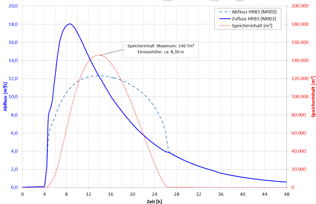
Abbildung 8-12 Variante 2: Ganglinien der Speichersimulation M003 – Becken oh. Rohda
