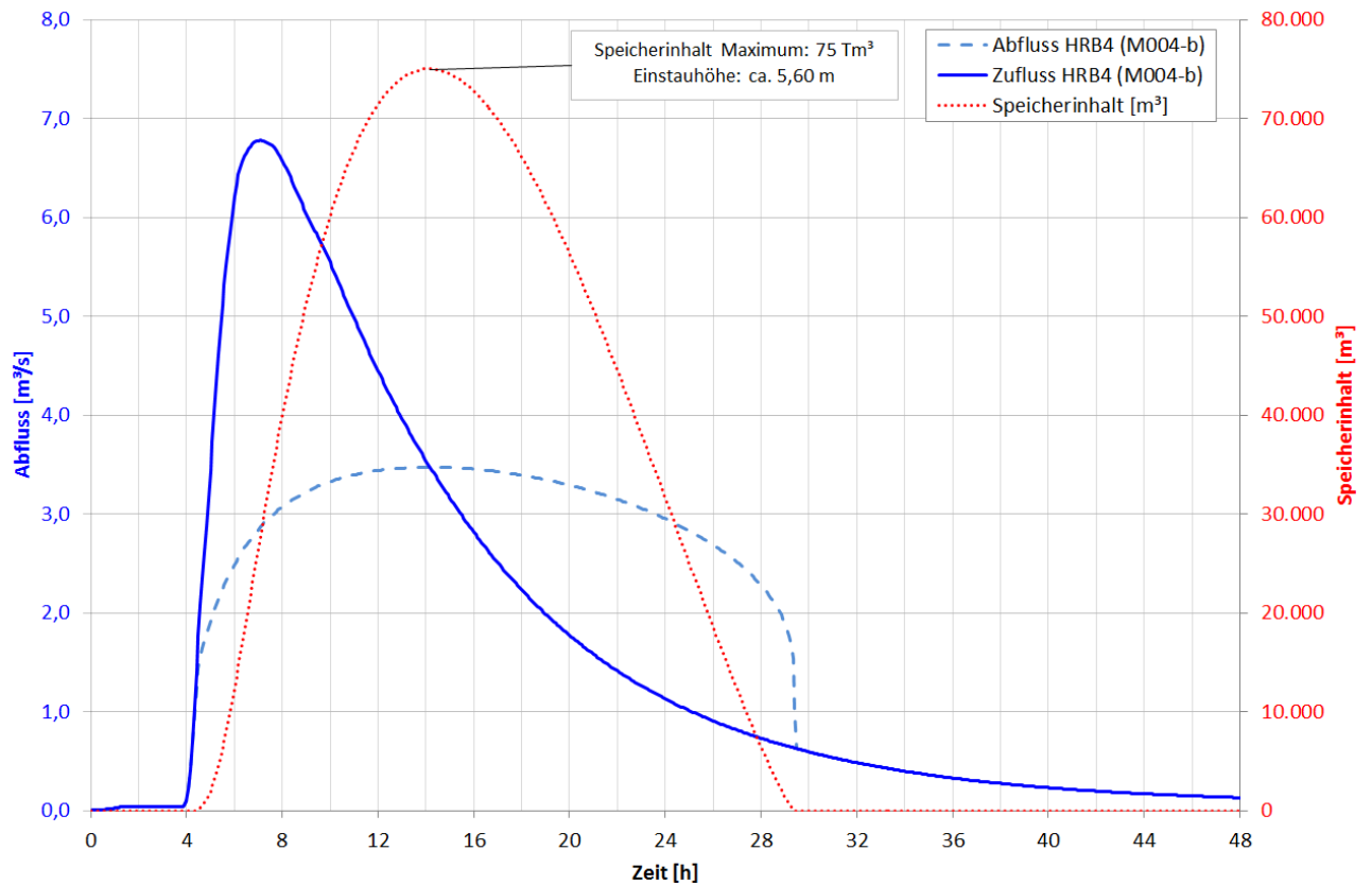
Abbildung 8-15 Variante 3: Ganglinien der Speichersimulation
