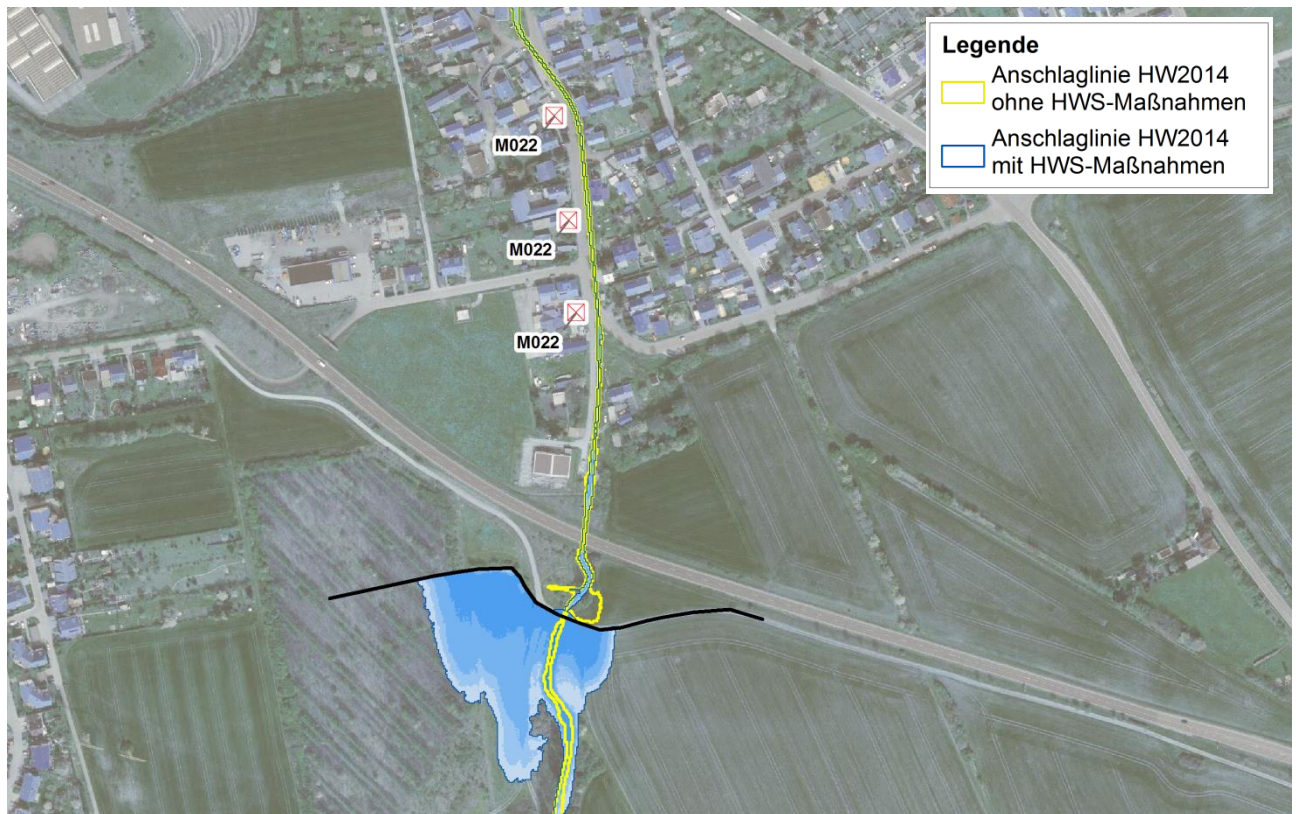
Abbildung 8-20 HW 2014 mit Hochwasserschutzmaßnahmen, Niedernissa
