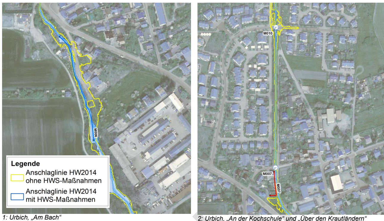
Abbildung 8-21 HW 2014 mit Hochwasserschutzmaßnahmen, Urbich
