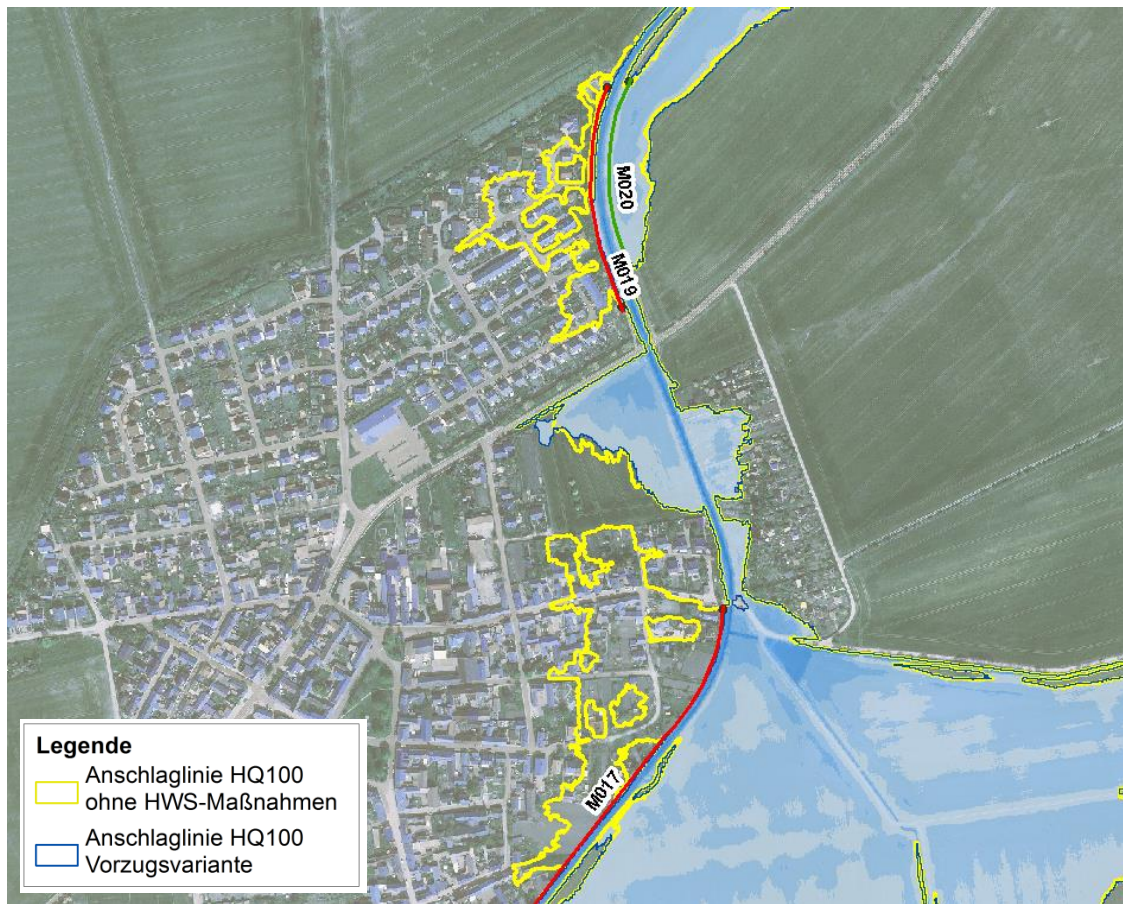
Abbildung 8-6 Ortslage Kerspleben - Auswirkungen der Maßnahmen M016, M017, M019 und M020
