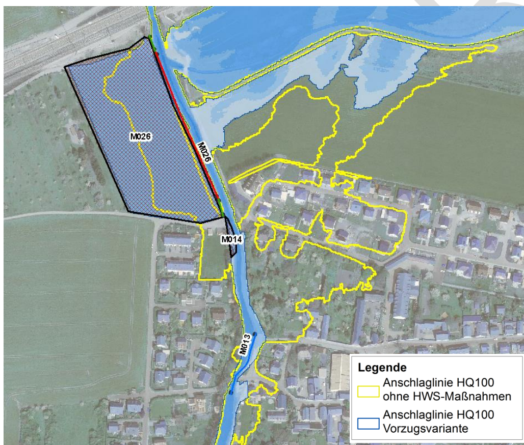
Abbildung 8-5 Ortslage Linderbach - Auswirkungen der Maßnahmen M013, M014 und M026
