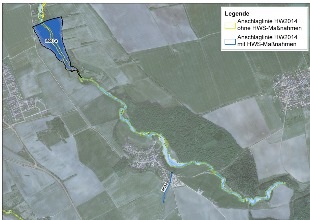
Abbildung 8-16 HW 2014 mit Hochwasserschutzmaßnahmen, oberhalb Büßleben
