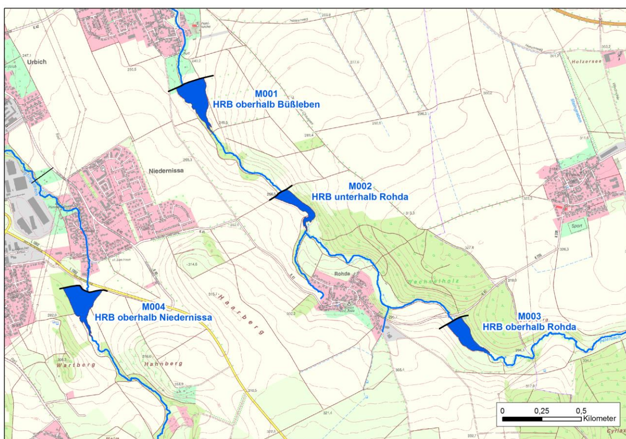
Abbildung 8-10 Potentielle Standorte für Hochwasserrückhalt im Einzugsgebiet
