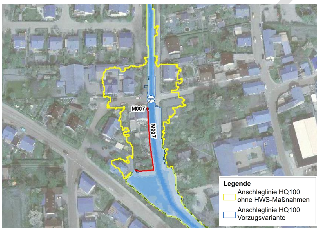
Abbildung 8-4 Auswirkungen der Maßnahme M007 in Urbich
