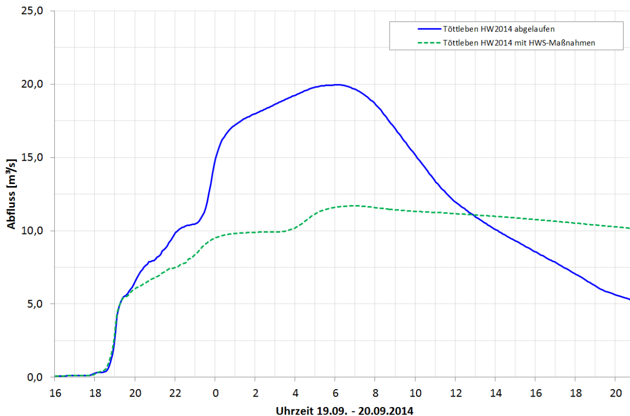
Abbildung 8-24 HW 2014 Abflussganglinie Töttleben - abgelaufen und prognostiziert
