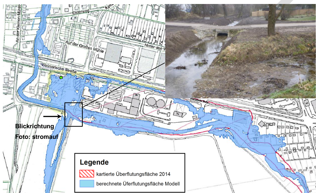
Abbildung 7-6 Linderbach Weimarische Straße, Hochwasser 2014 – Vergleich Kalibrierungsergebnis
