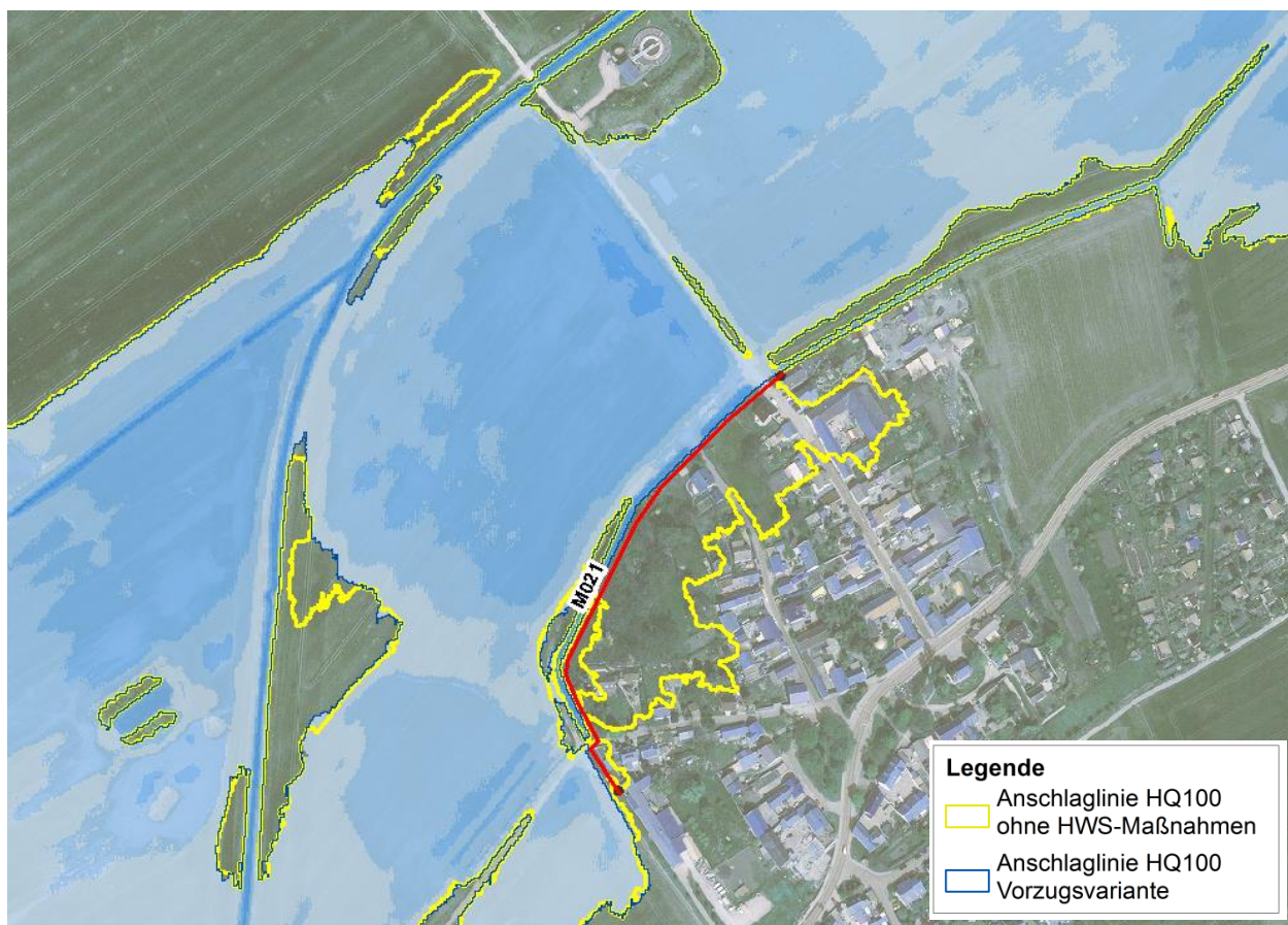
Abbildung 8-7 Ortslage Töttleben - Auswirkungen der Maßnahmen M016, M017, M019 und M020
